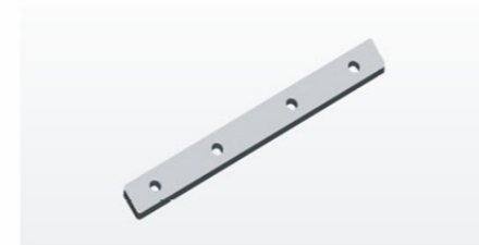
名称/Name: 一字连接件 Straight connector 材质/Material: 铝材/Aluminum 颜色/Colour: 砂白、砂黑/White、Black 尺寸/Size: 100x9.7x2.5mm
